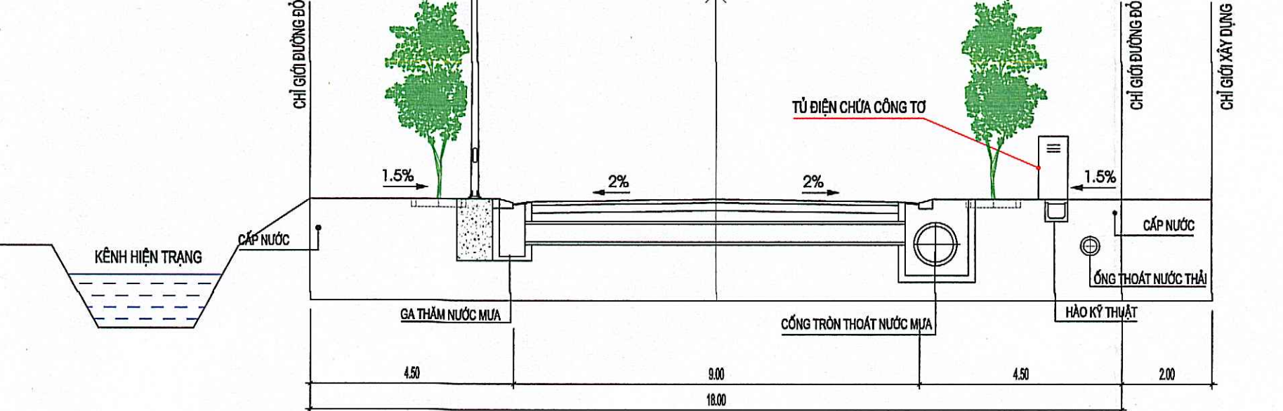
MẶT CẮT TỔNG HỢP KỸ THUẬT 2-2
