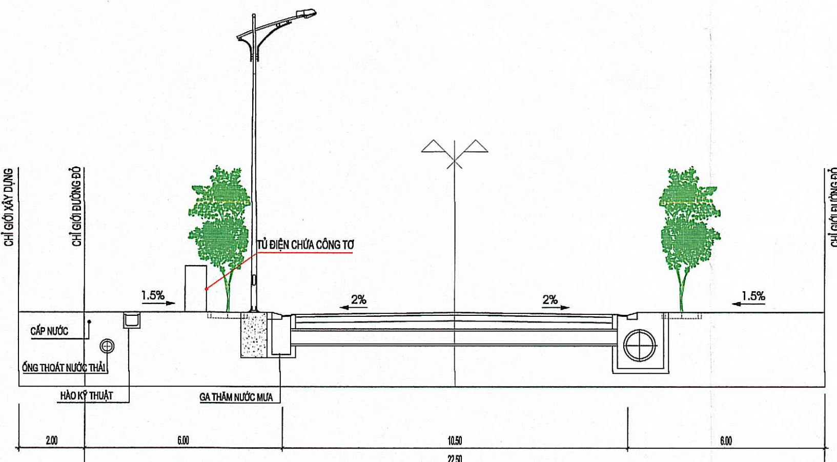
MẶT CẮT TỔNG HỢP KỸ THUẬT 1-1
