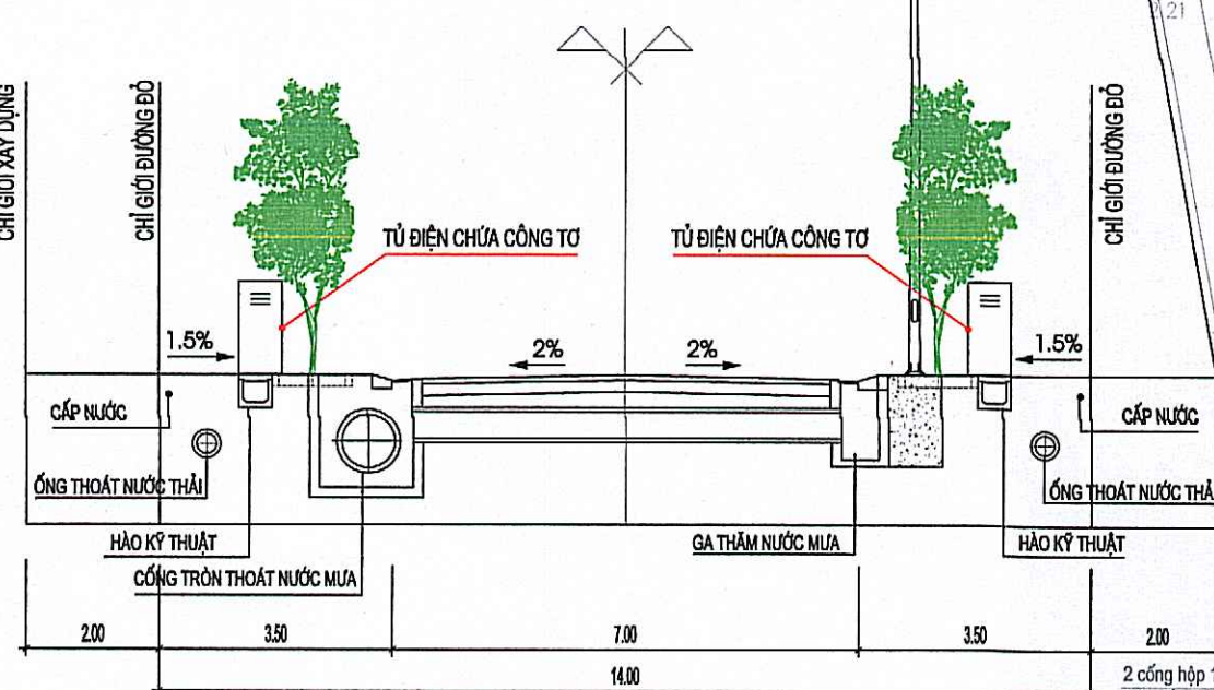
MẶT CẮT TỔNG HỢP KỸ THUẬT 3-3
