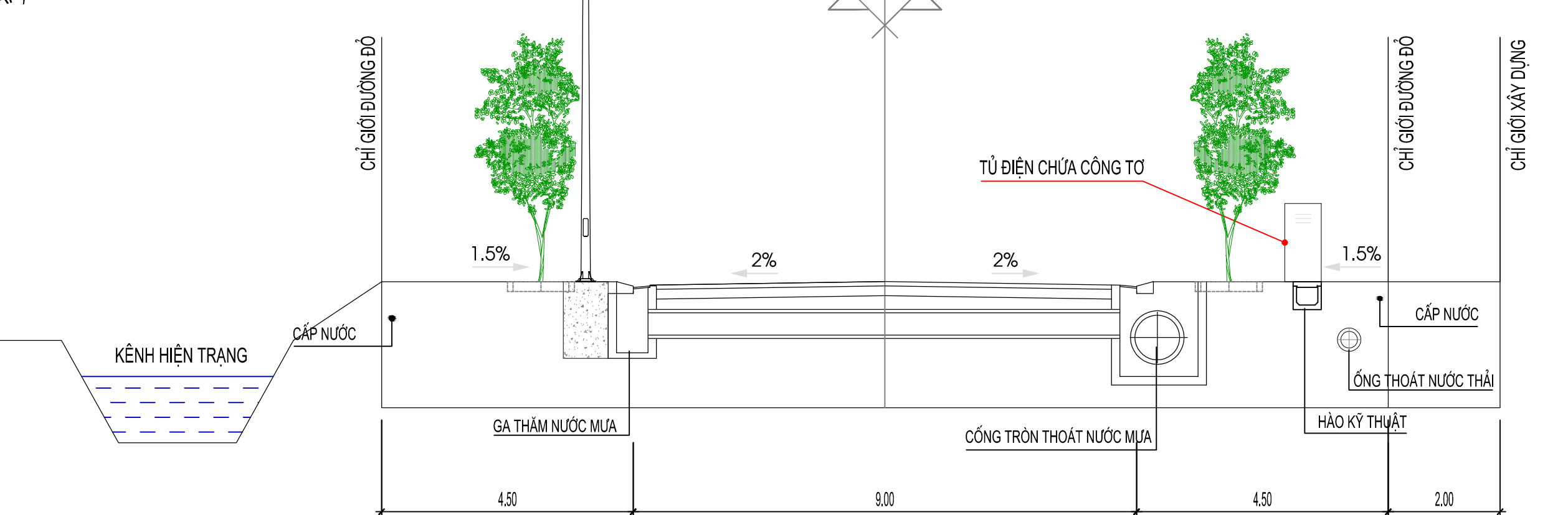
MẶT CẮT TỔNG HỢP KỸ THUẬT 2-2
