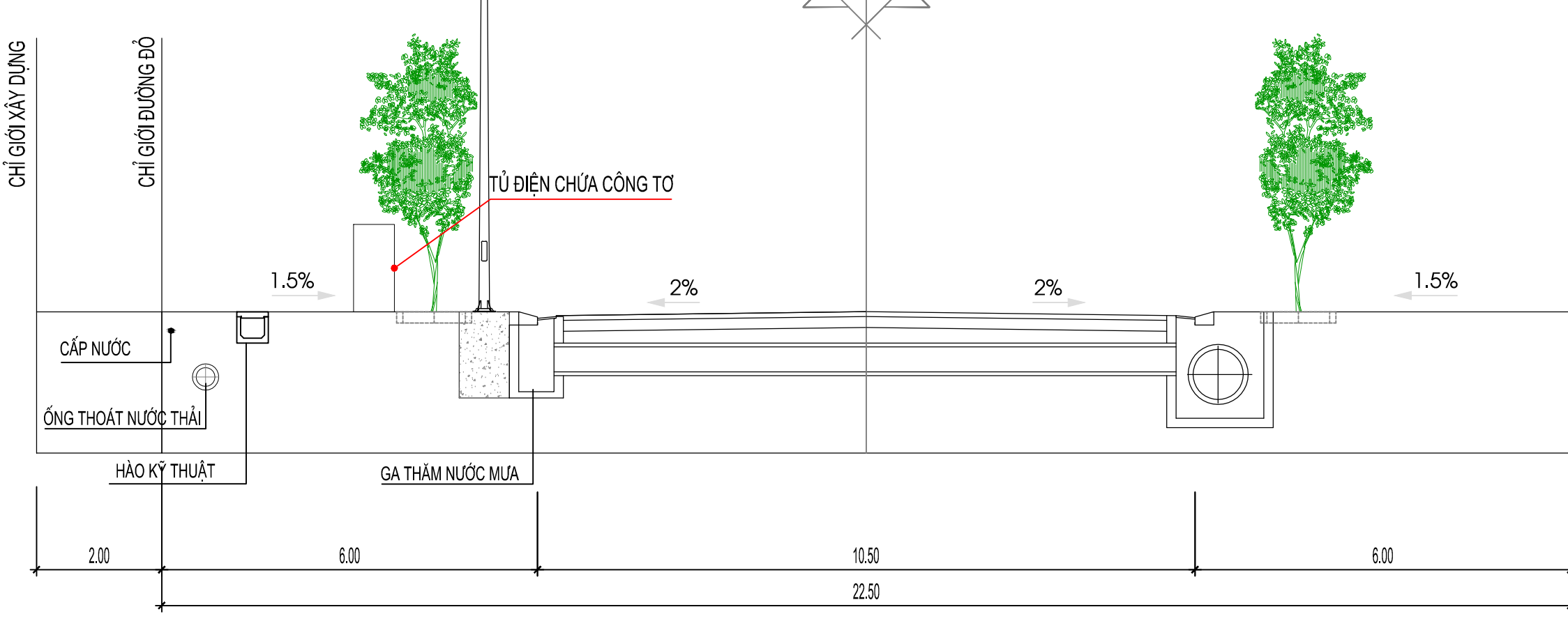
MẶT CẮT TỔNG HỢP KỸ THUẬT 1-1
