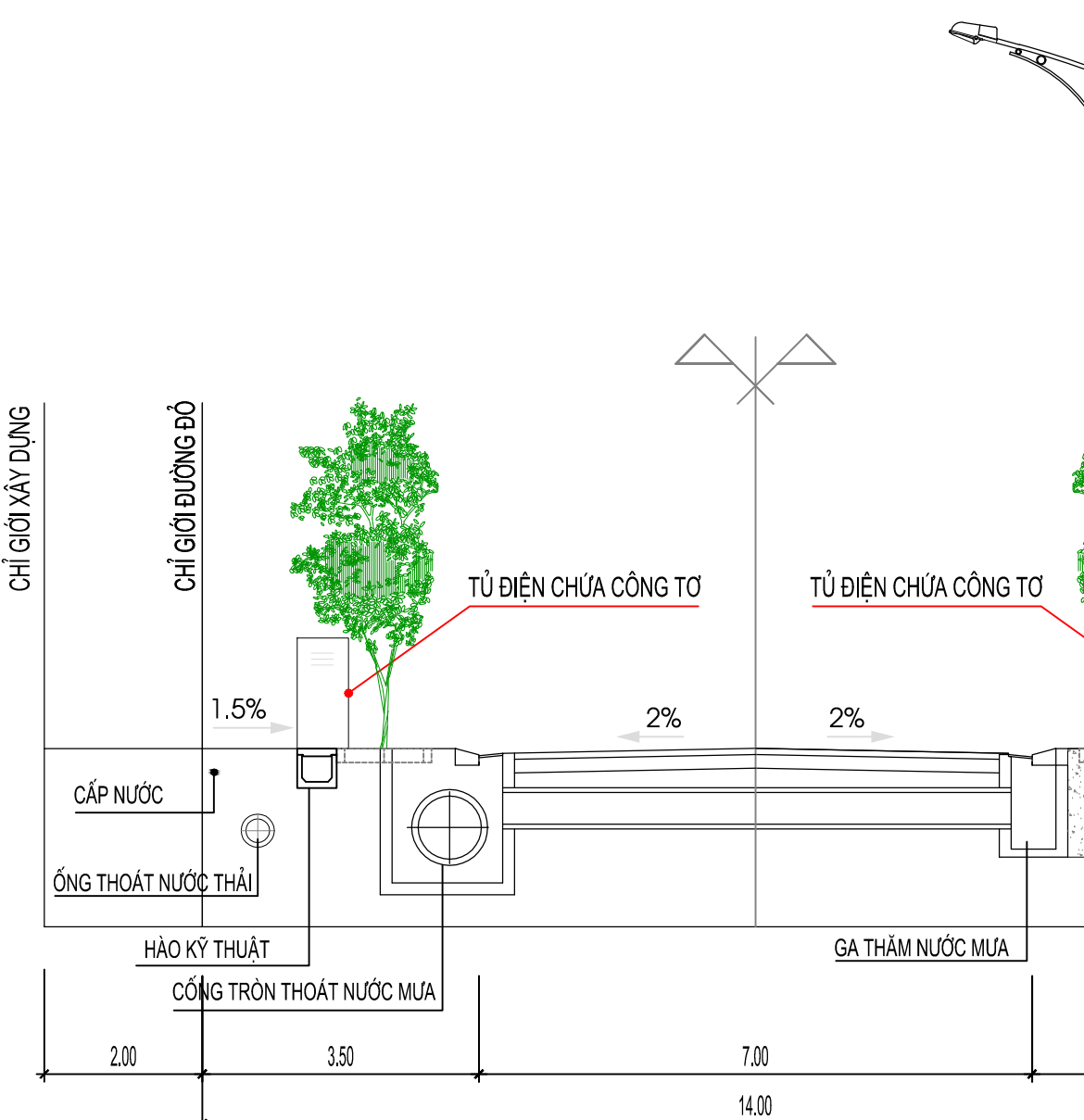
MẶT CẮT TỔNG HỢP KỸ THUẬT 3-3
